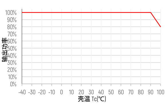
输出功率vs. 壳温
